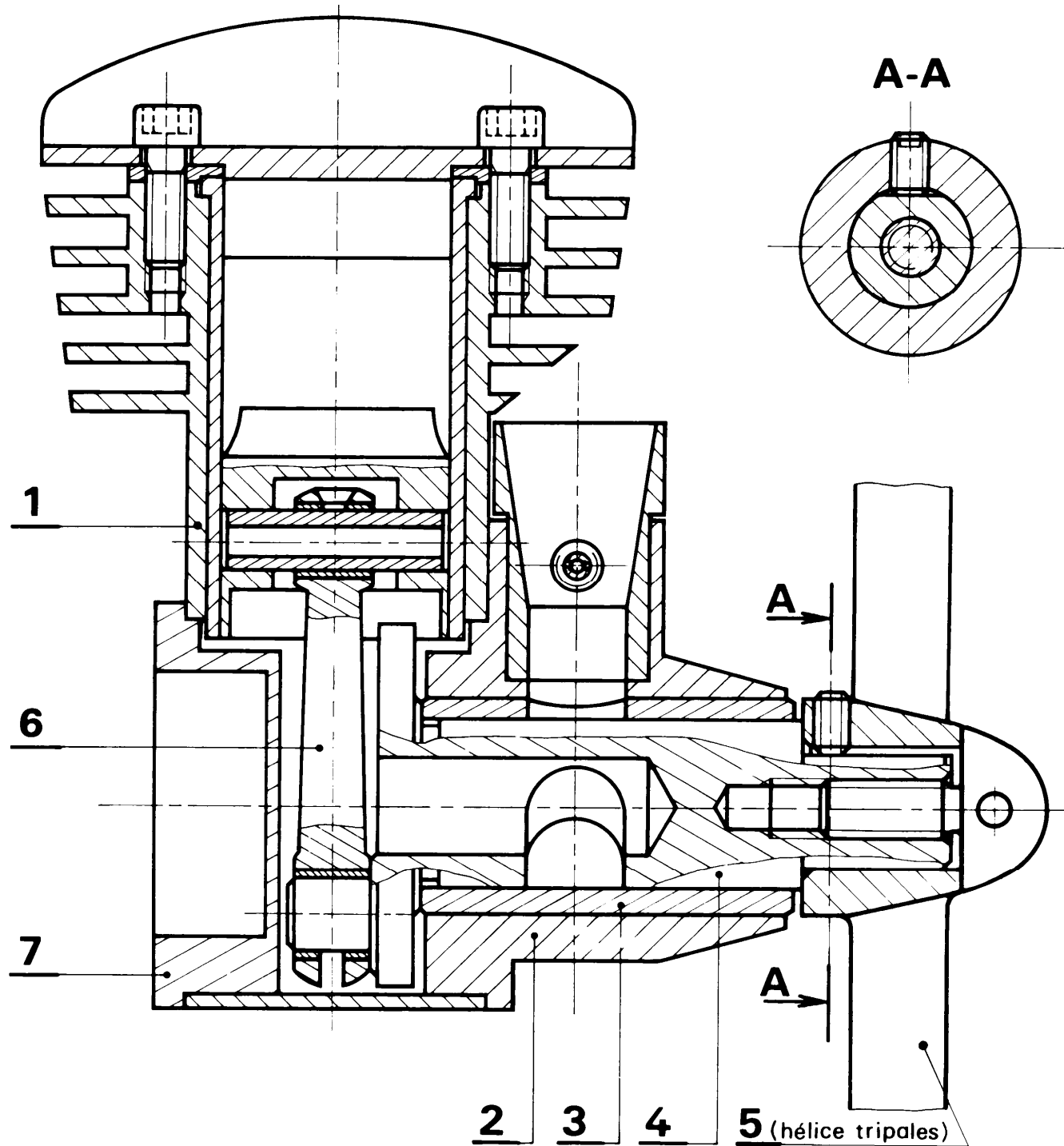
PLAN D'ENSEMBLE DU MICROMOTEUR
