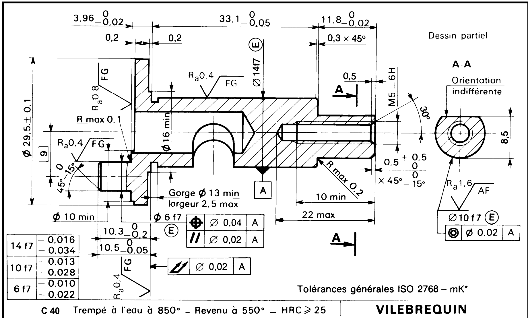
PLAN DE DEFINITION DU VILEBREQUIN
